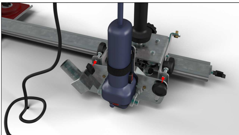
Fig. 6.4.11 Avvitare i due bulloni e ruotare i due pomelli.
