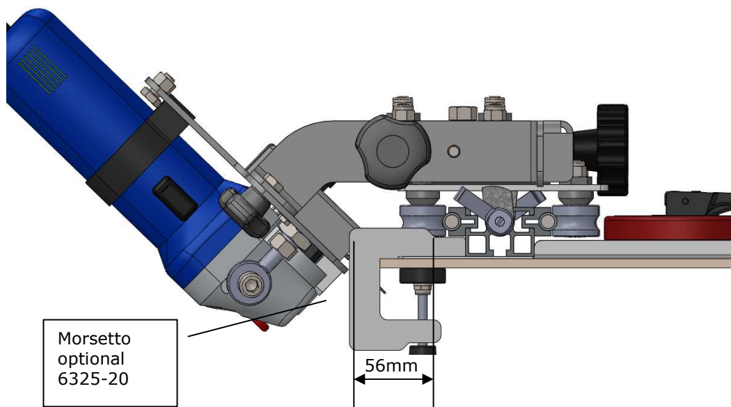
Fig. 6.3.3 Taglio 45° (Jolly) posizione morsetto distanziatore
