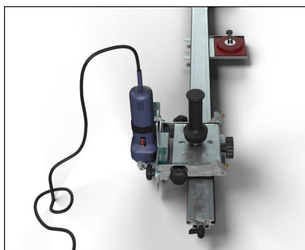
Fig. 6.3.1 Taglio lineare.
