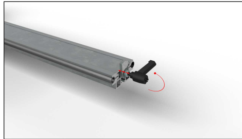
Fig.6.4.9 Ruotare vite di fissaggio guide.
