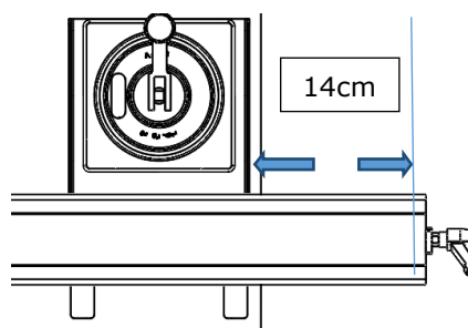
Fig.6.3.1.1 misura della guida dalla piastrella
