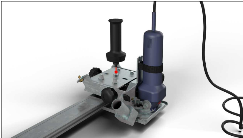
Fig. 6.4.10 Pomello di bloccaggio della regolazione millimetrica.
