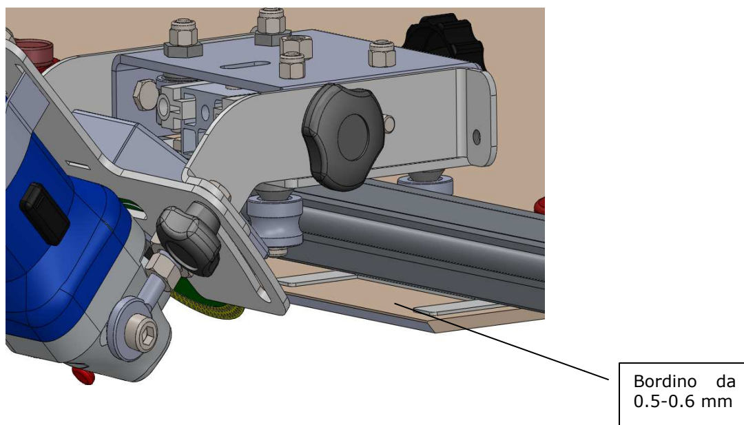
Fig. 6.3.4 Taglio 45° (Jolly)
