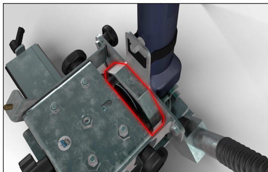
Fig. 3.1 Protezione fissa del disco da taglio.
