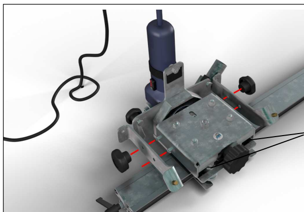
Fig.6.4.7 Svitare i pomelli, ruotare di 180° le due staffe e avvitarle i pomelli.
