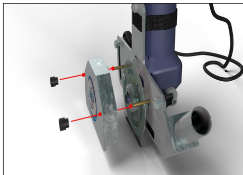
Fig. 3.1.1 Fissaggio protezione con viti.
