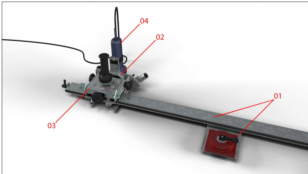
Fig. 2.1 Componenti della macchina.
