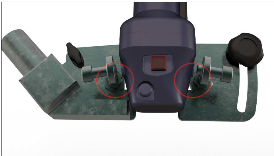
Fig. 6.4.6 Due viti regolabili in base alle dimensioni della smerigliatrice. Regolare la misura e stringere i bulloni solo nel caso in cui la smerigliatrice non sia del tipo Bosch GWS 7-115
